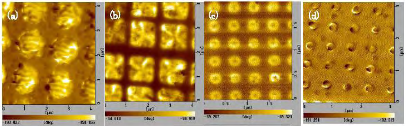
図3.14 微細ドットの磁気構造 (a) 縞状磁区(Co 円形ドット 1.2\mu\text{m}\phi ), (b) 環流磁区(パーマロイ正方形ドット 1.2\mu\text{m} ), (c) ボルテックス(パーマロイ円形ドット 300\text{nm}\phi ), (d) 単磁区(Co 円形ドット 100\text{nm}\phi )
