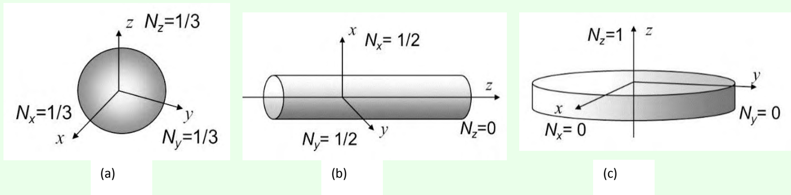
図3.6 反磁界係数は磁性体の形と向きで異なる。
