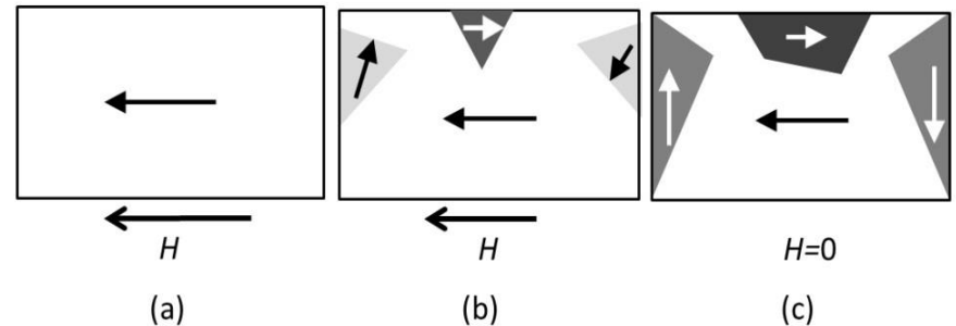
図3.28 磁気飽和状態から磁界を減らしていくと、さまざまな磁化方向の磁区が核発生し、成長するが、もとの状態には戻れない。
