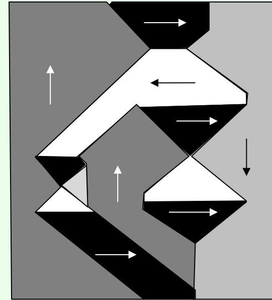
図3.2 磁化前の磁性体の磁区構造の模式図
