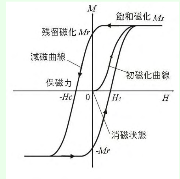
図3.15 強磁性体の典型的な磁化曲線
