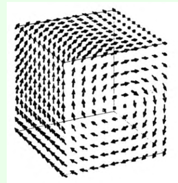
図3.13 ボルテックス構造
