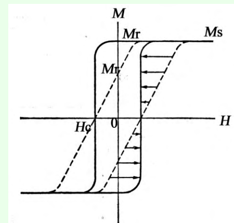
図3.7 測定した磁化曲線は図の点線のように傾いているが、磁気モーメントに加わる磁界が反磁界の分だけ減少しているため、適切な補正を行うと実線のようになる。
