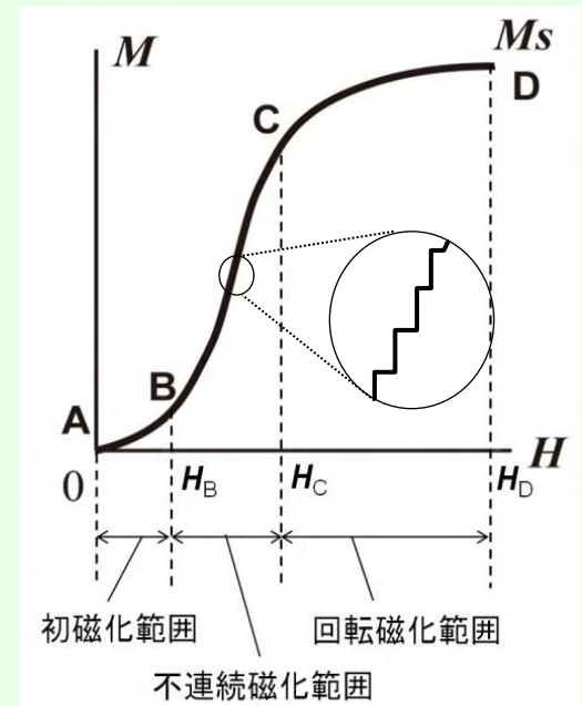
図3.18 初磁化曲線
