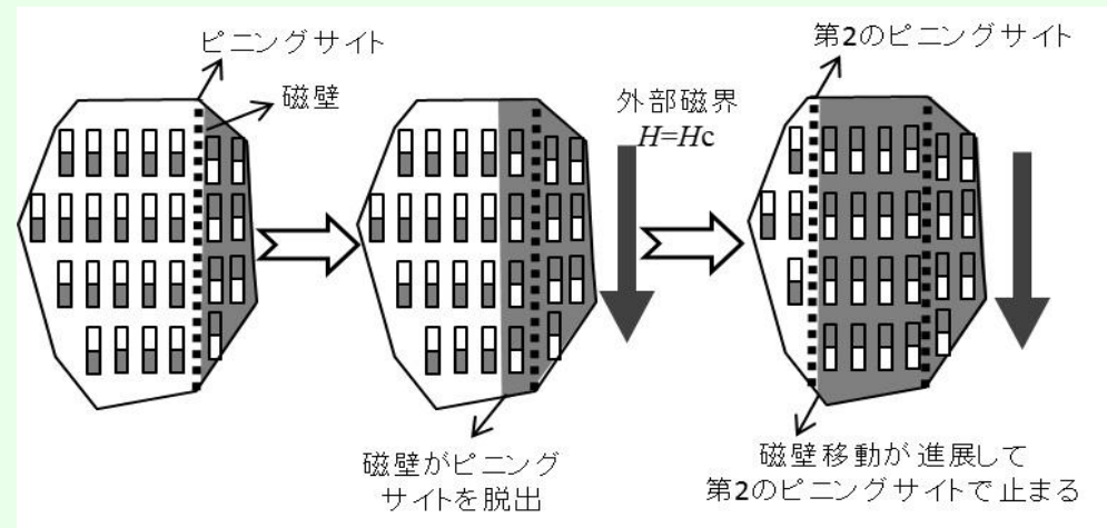
図3.27 ピニング型磁性体の反転機構の模式図
