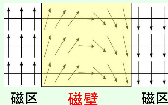
図3.11 磁壁内では原子磁石が徐々に回転して隣り合う磁区の磁化をつなぐ
