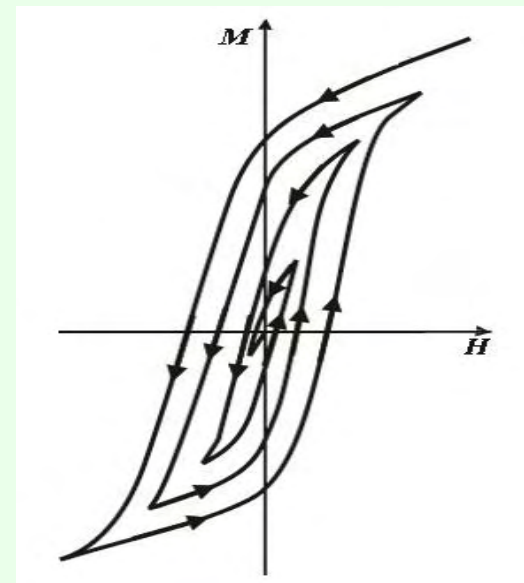
図3.20 交流消磁の消磁過程
