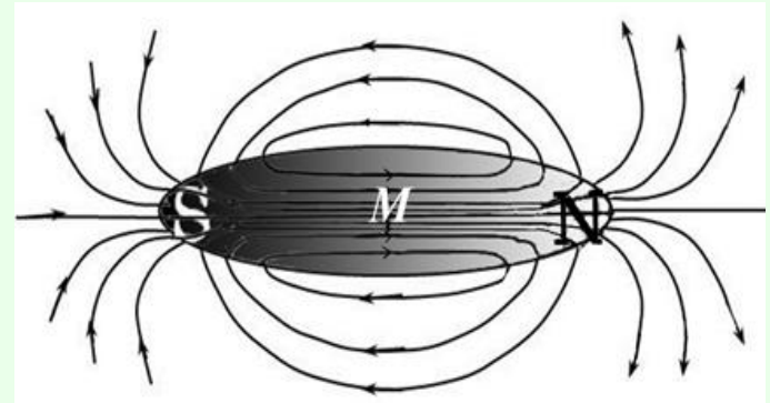
図3.4 磁束線は磁化と連続
