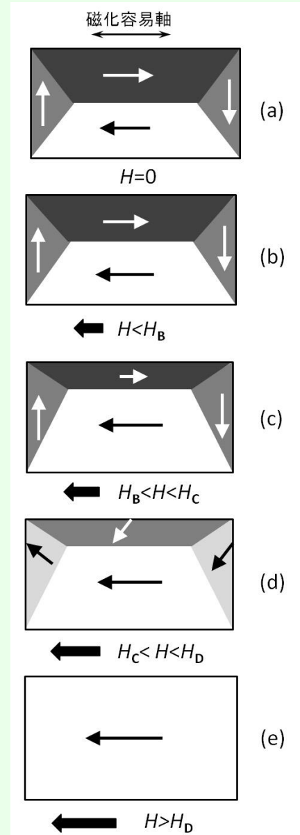
図3.19 初磁化曲線の磁壁移動・磁化回転による説明
