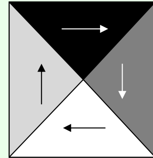
図3.12 環流磁区構造
