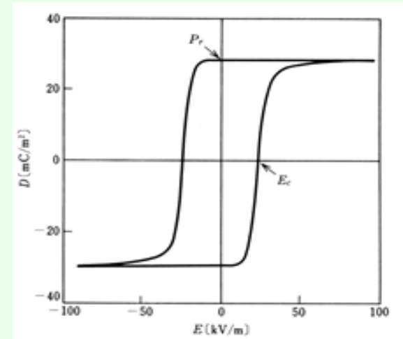
図3.16 強誘電体硫酸グリシンのD-Eヒステリシス曲線(佐藤勝昭編著：応用物性(オーム社1991)p.134による)
