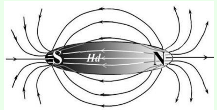
図3.5 磁力線はN極からS極に向かって流れている
