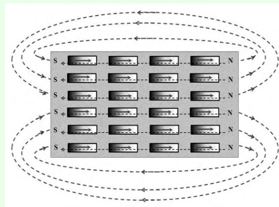
図3.8 磁性体内部の原子磁石は反磁界を受けて静磁的に不安定
