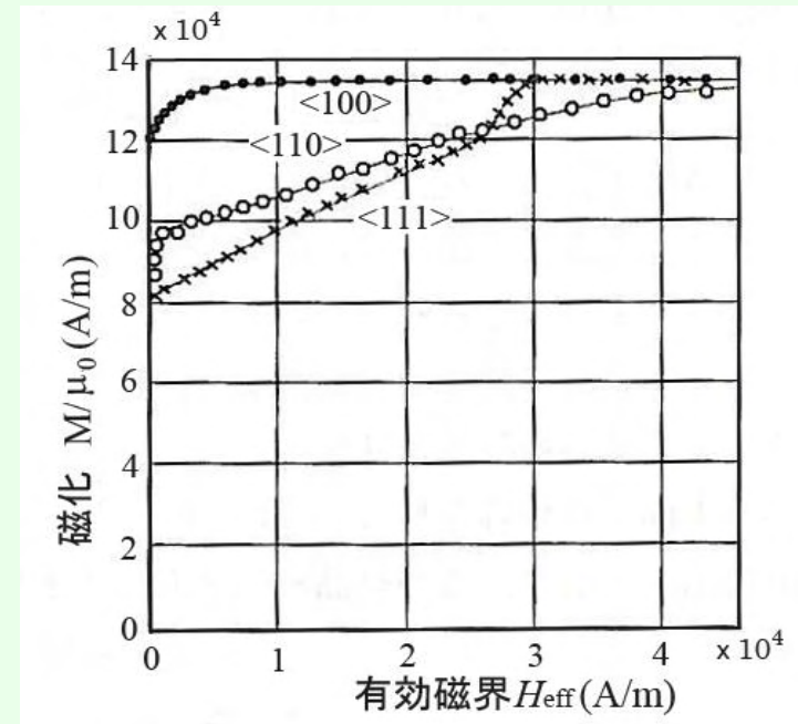
図3.21 Feの磁化曲線の結晶方位依存性(Kayaによる。佐藤勝昭編著:応用物性p.209)
