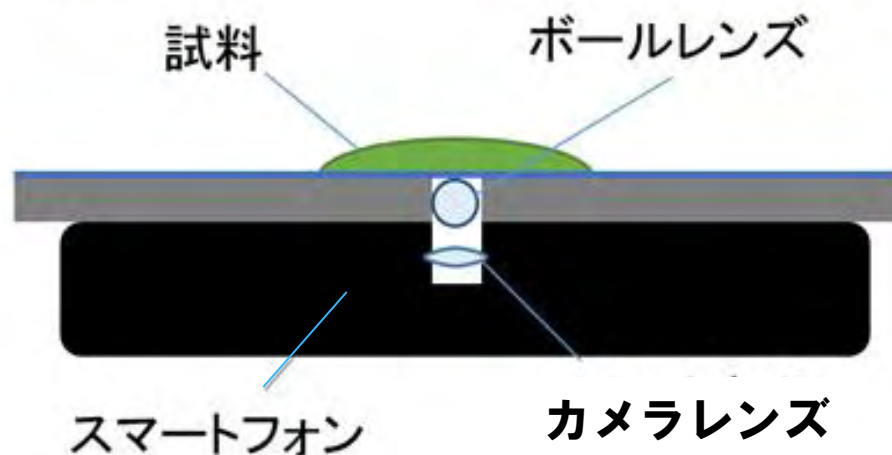
b. 側面図
